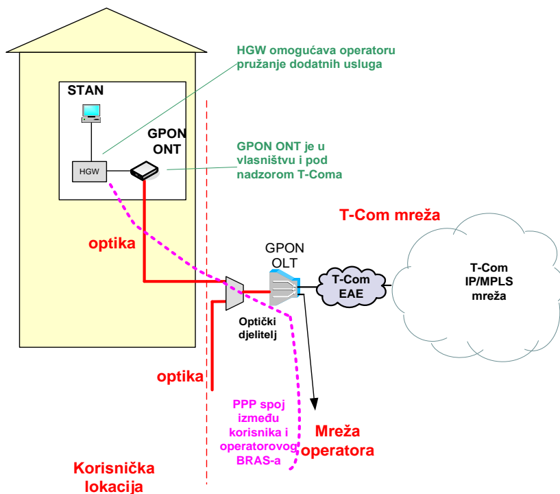
Slika 6. Način realizacije usluge veleprodajnog širokopojasnog pristupa za Internet uslugu na temelju FTTH rješenja na OLT razini
